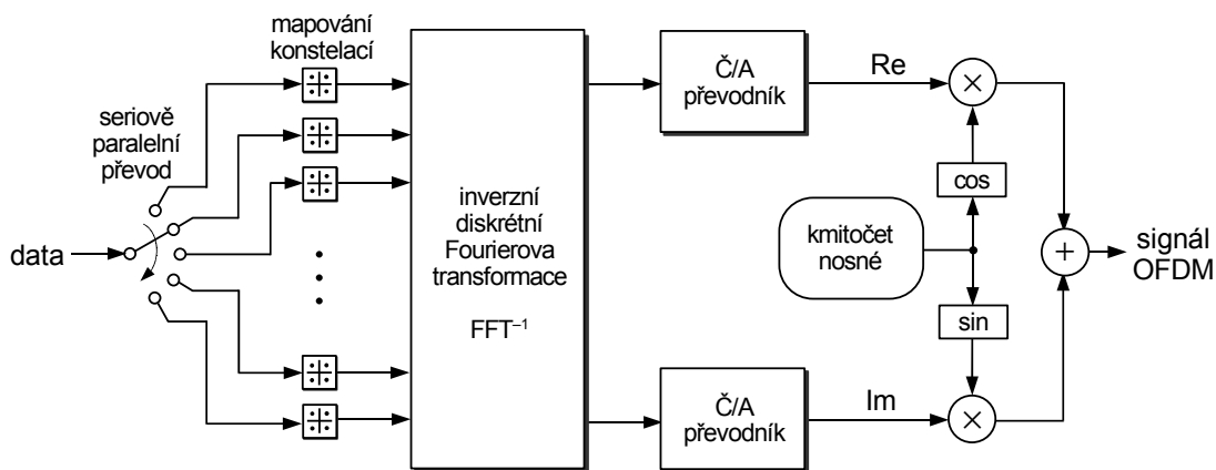
Obrázek 10.14.: Modulátor OFDM využívající rychlou Fourierovu transformaci ( \text{FFT}^{-1} ) pro vytvoření množství modulovaných nosných.
