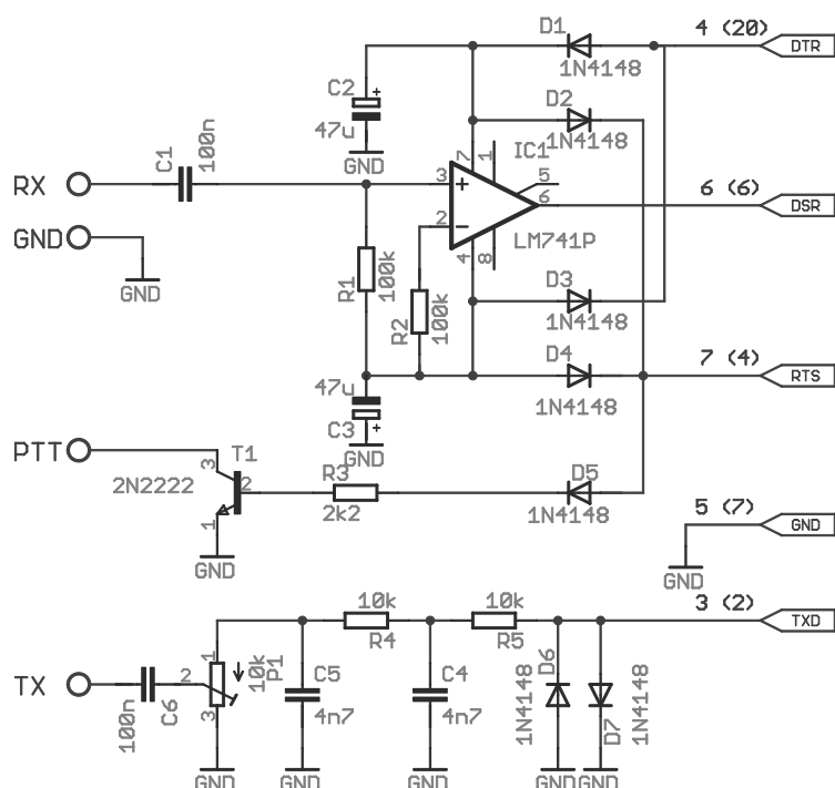
Obrázek 7.14.: Schéma interfejsu Hamcomm.
