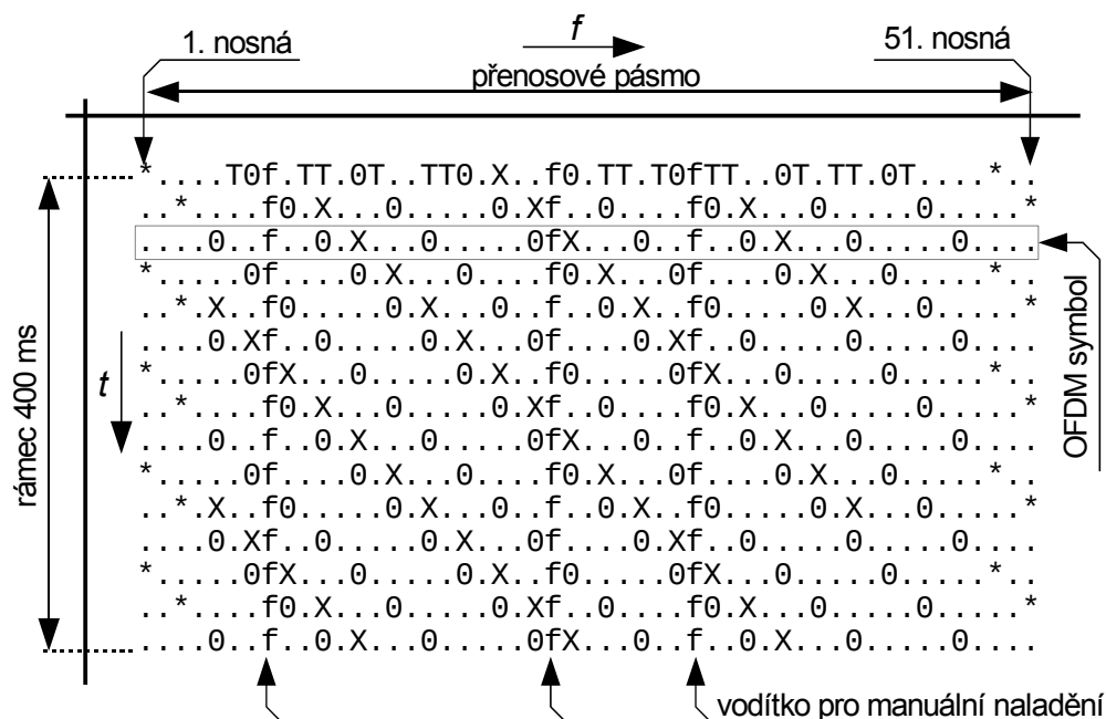
Obrázek 10.9.: Příklad složení jednoho rámce pro Mode B , pásmo 2,5 kHz. Legenda: . – MSC buňka, X – FAC buňka, T – časové vodítka, f – ladící vodítka, 0 – rozptýlená a * – posílená ladící vodítka pro synchronizaci.
