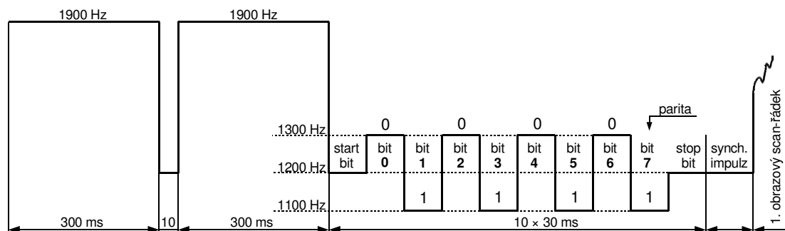
Obrázek 3.11.: Struktura VIS kódu s hodnotou 42.
