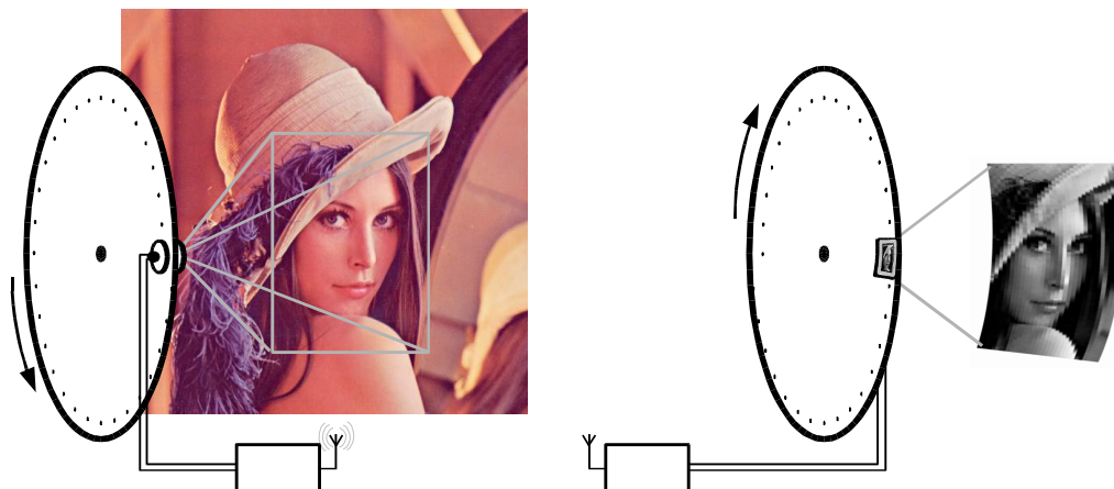
Obrázek 13.2.: Bairdova televizní soustava s Nipkowovým diskem.
