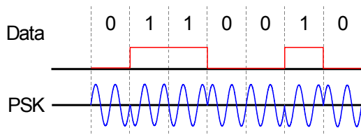
Obrázek 10.1.: Digitální modulace BPSK – dvoufázové klíčování fázovým posuvem.
