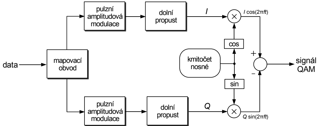
Obrázek 10.10.: Modulátor QAM.
