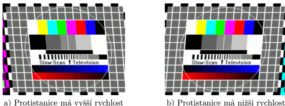
Obrázek 7.9.: Sešikmení obrazu při rozdílných rychlostech rozkladu.
