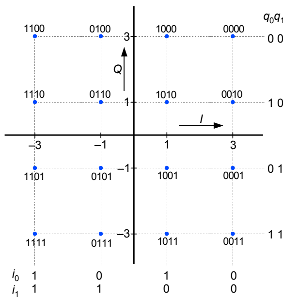
Obrázek 10.11.: Konstelační diagram pro QAM-16 s pořadím bitů \{i_0, i_1, q_0, q_1\} použitým v DRM.
