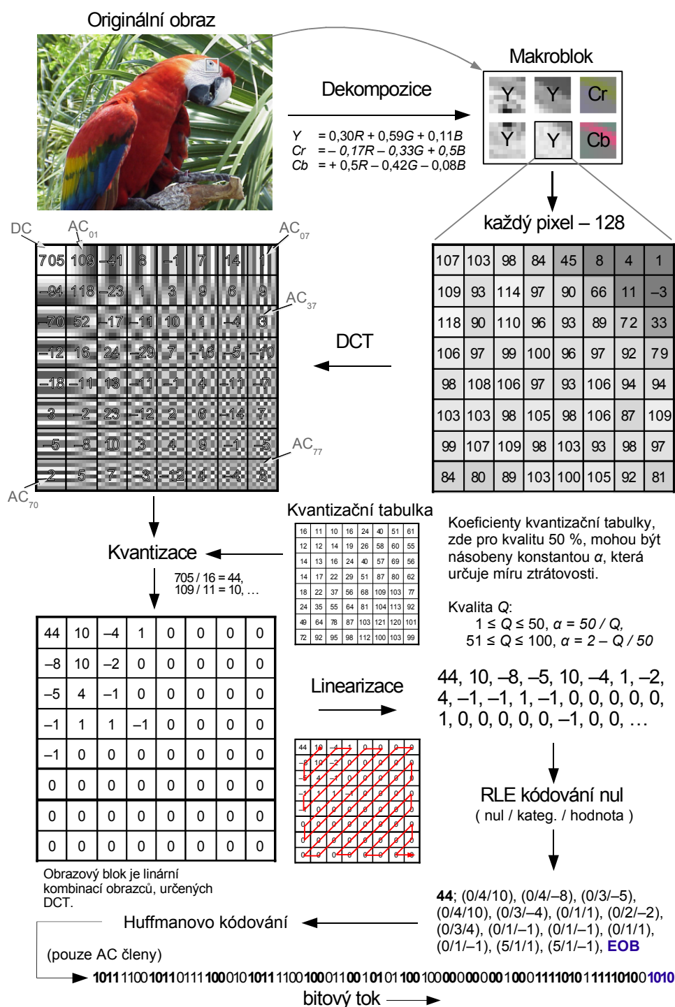
Obrázek 9.3.: JPEG komprese pro jeden jasový blok 8×8.
